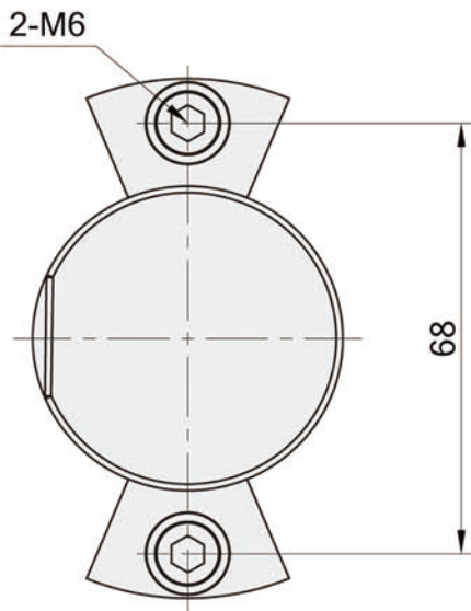
徑向入水
